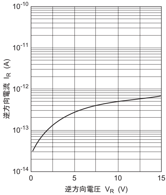
图1. 逆方向特性
