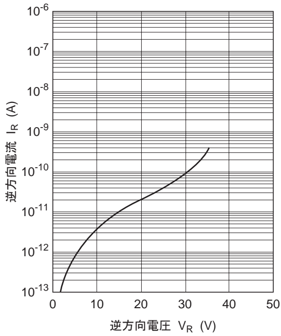
图1. 逆方向特性
