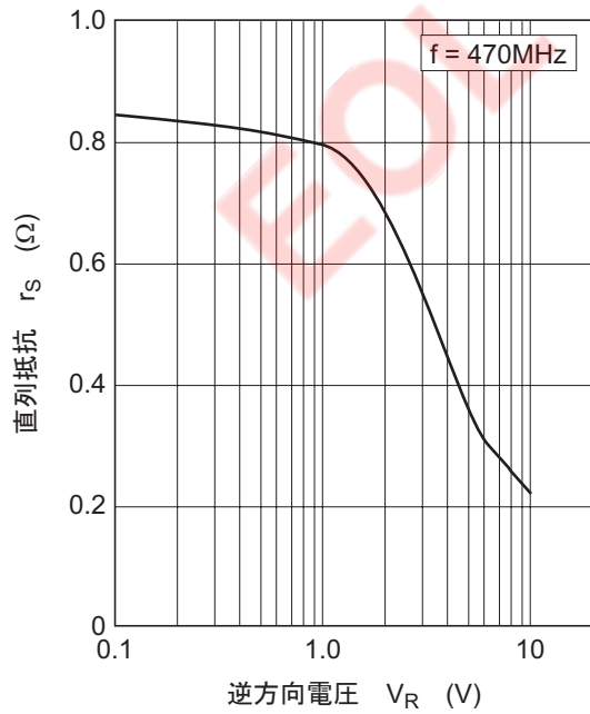
图3. 直列抵抗 对 逆电压特性
