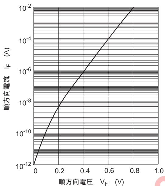
图1. 顺方向特性
