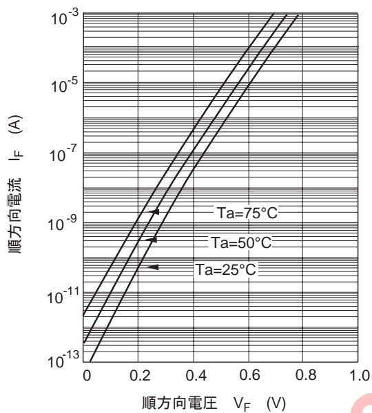
图1. 顺方向特性
