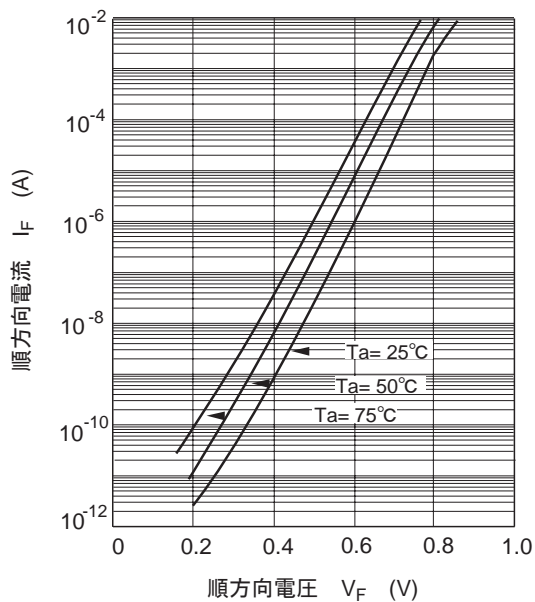
图1. 顺方向特性
