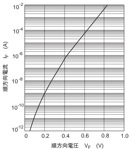
图1. 顺方向特性
