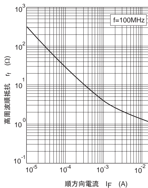
图4. 高周波顺抵抗 对 顺电流特性
