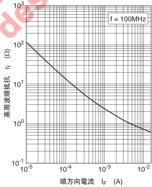
图4. 高周波顺抵抗 对 顺电流特性
