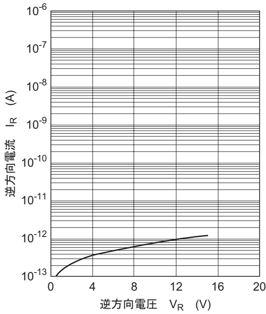
图1. 逆方向特性
