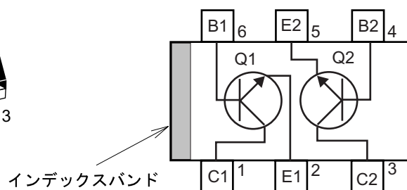
ピン配置図
