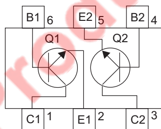
ピン配置
