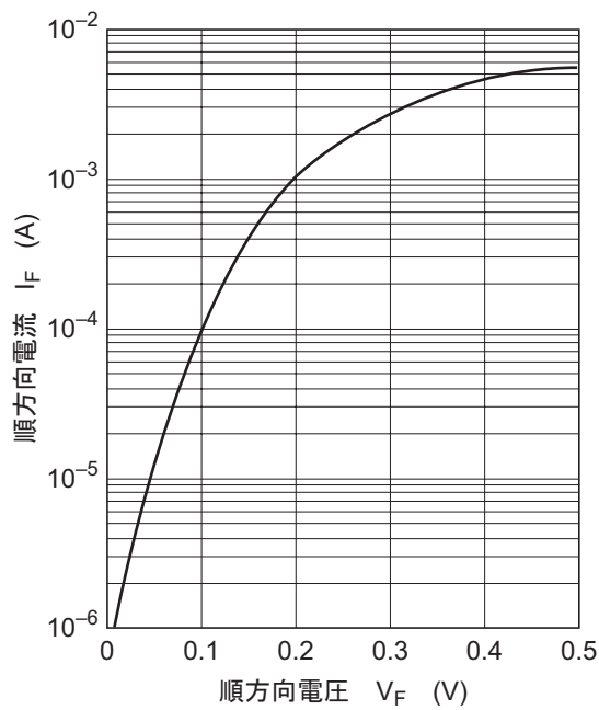
図1. 順方向特性
