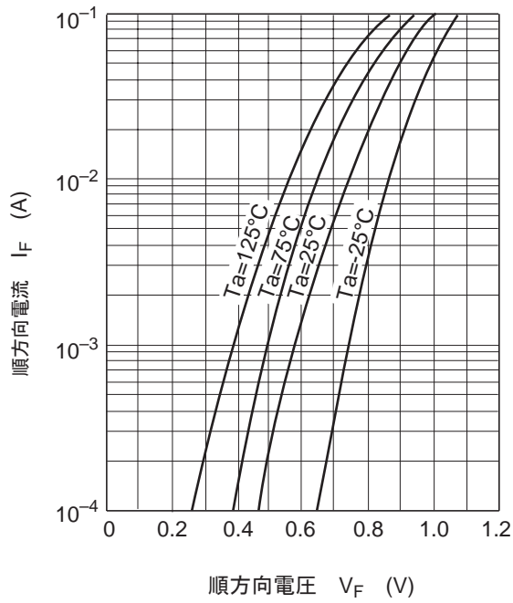
图1. 顺方向特性
