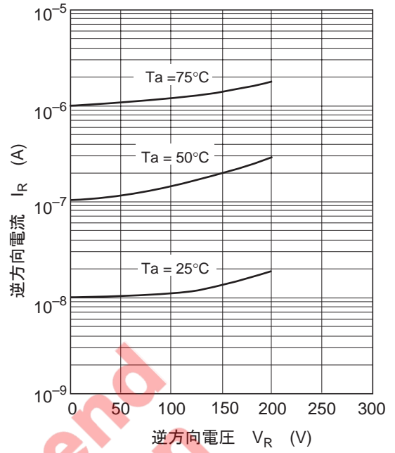
图2. 逆方向特性
