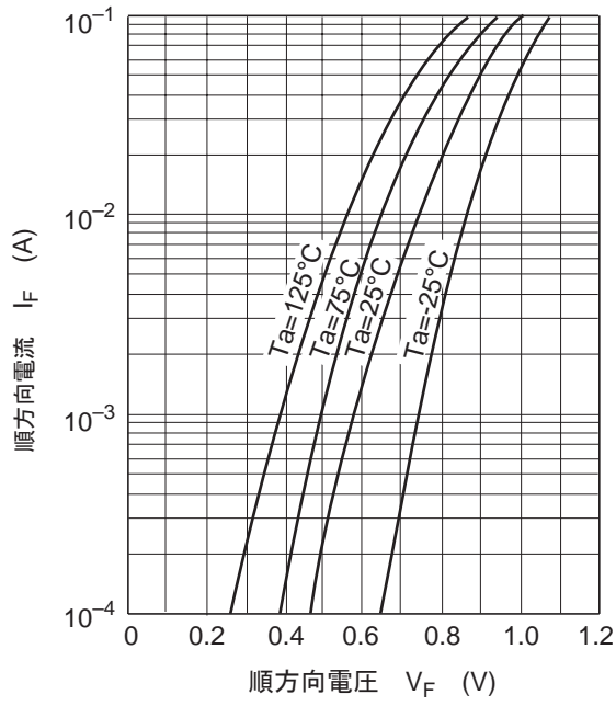
图1. 顺方向特性
