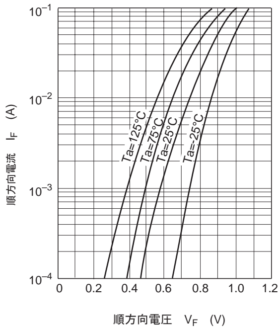
图1. 顺方向特性
