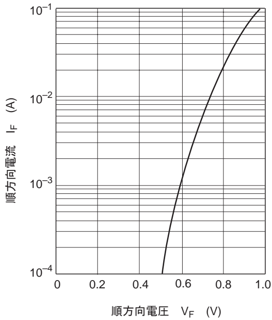
図1. 順方向特性
