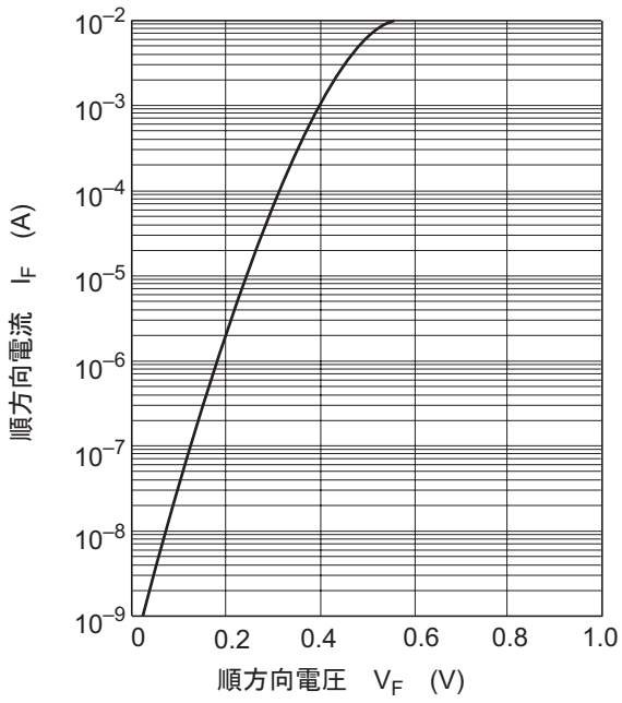
图1. 顺方向特性
