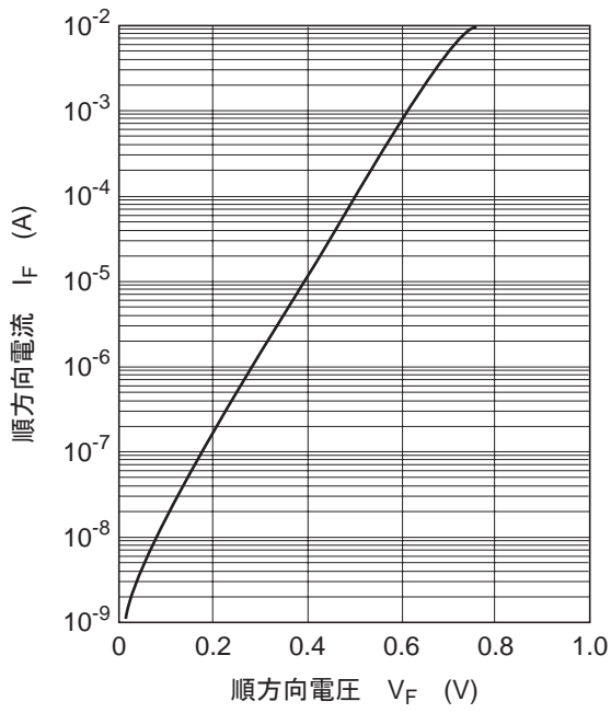
図1. 順方向特性
