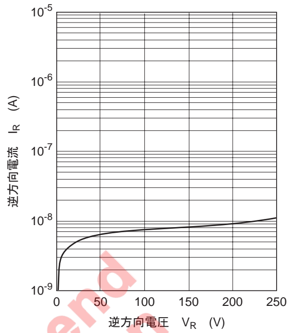
図2. 逆方向特性
