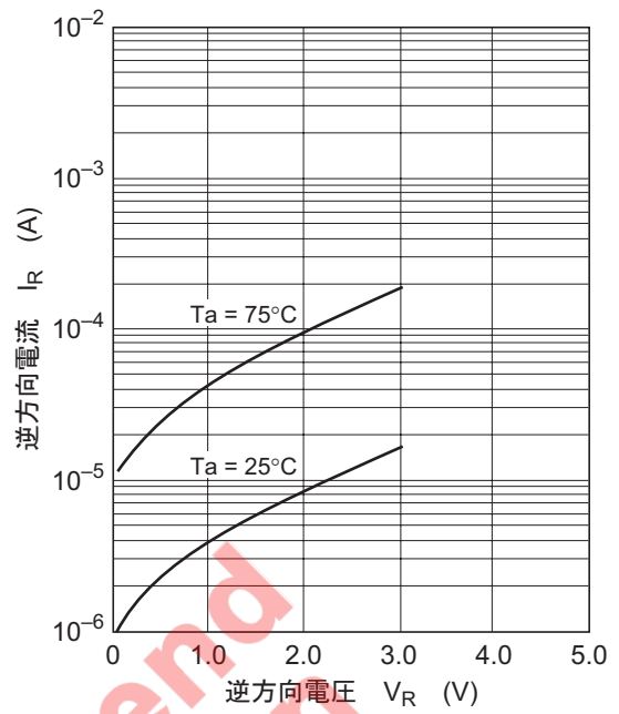
图2. 逆方向特性
