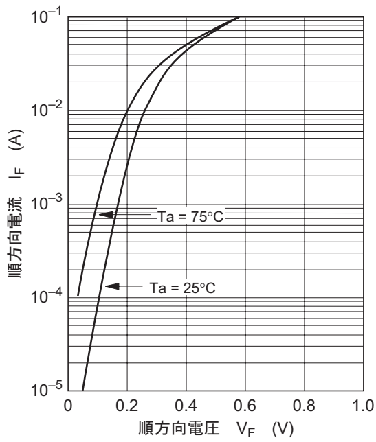
图1. 順方向特性
