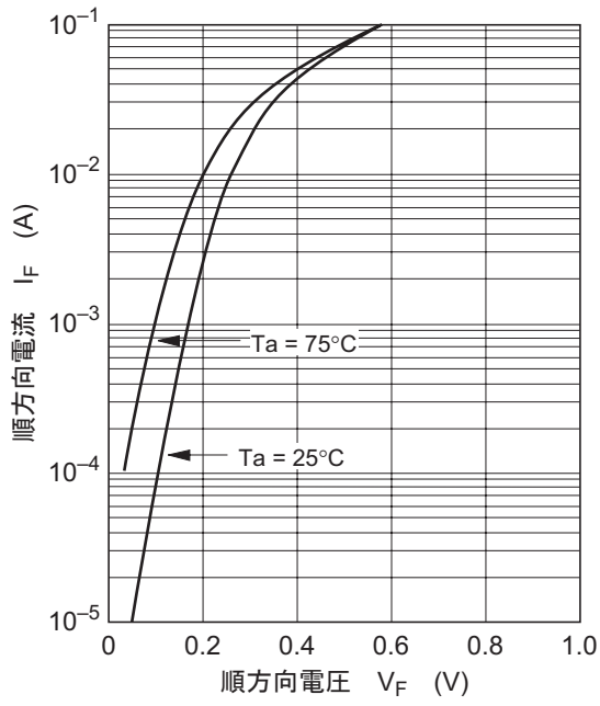
图1. 顺方向特性
