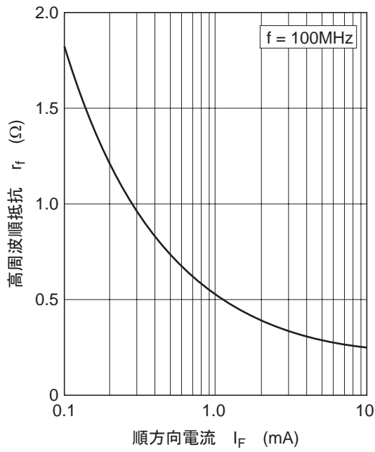
图1. 高周波順抵抗 对 順電流特性
