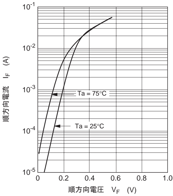
图1. 順方向特性
