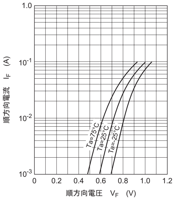
图1. 順方向特性
