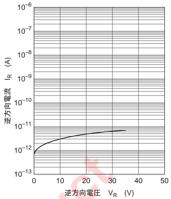
图2. 逆方向特性
