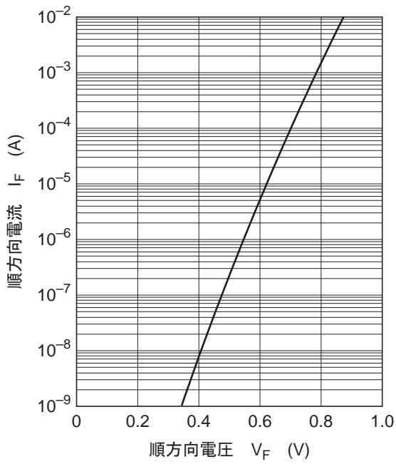
图1. 顺方向特性
