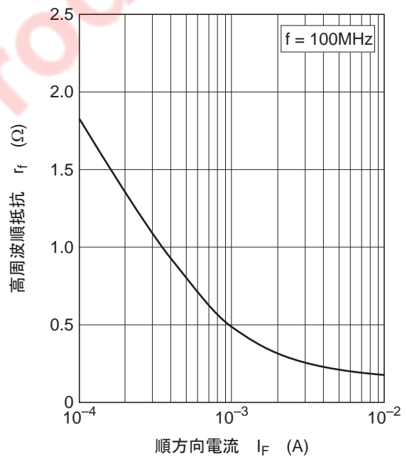
图4. 高周波顺抵抗 对 顺电流特性
