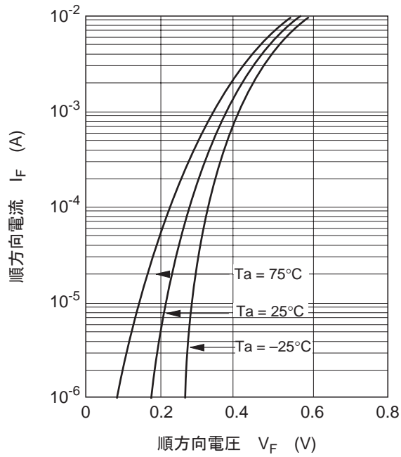
図1. 順方向特性
