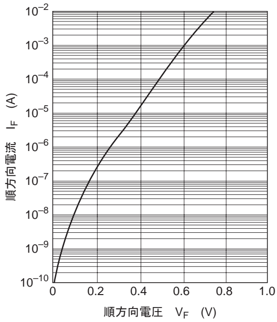
图1. 順方向特性
