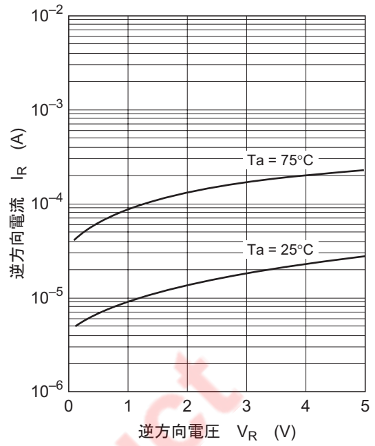
图2. 逆方向特性
