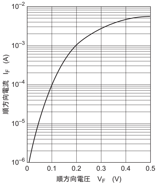
图1. 顺方向特性
