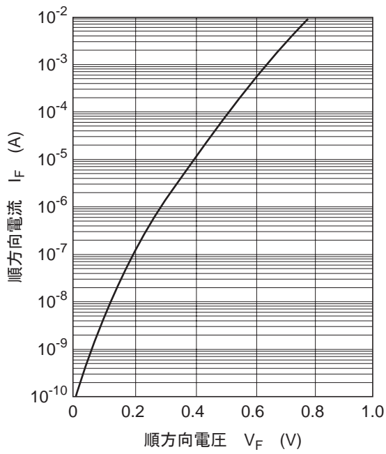
図1. 順方向特性
