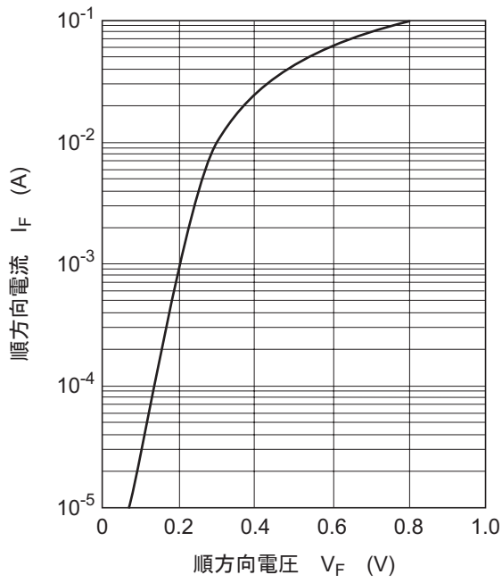
图1. 順方向特性
