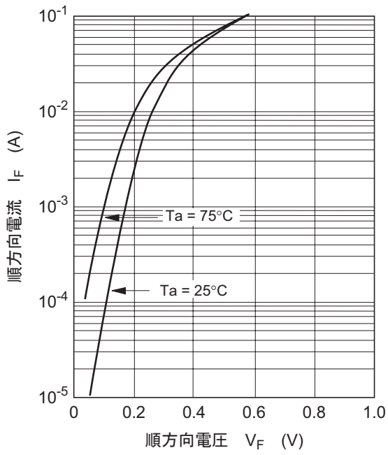
图1. 順方向特性
