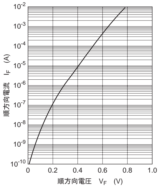
图1. 順方向特性
