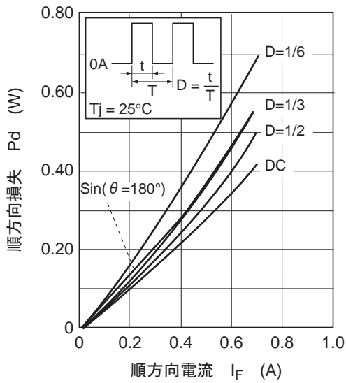
図4. 順方向損失 対 順電流特性
