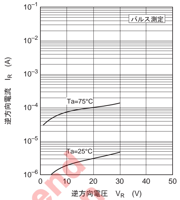
図2. 逆方向特性
