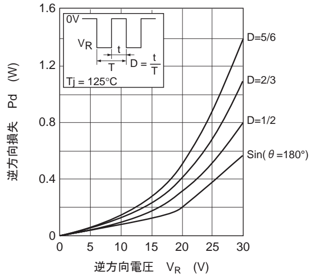
図5. 逆方向損失 対 逆電圧特性
