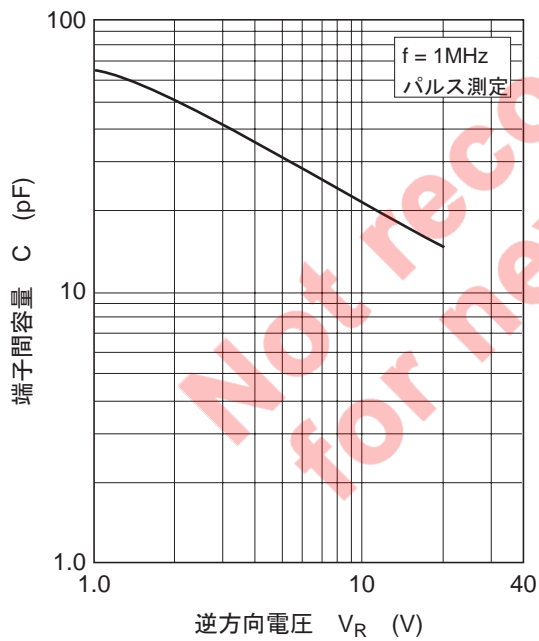
図3. 端子間容量 対 逆方向電圧
