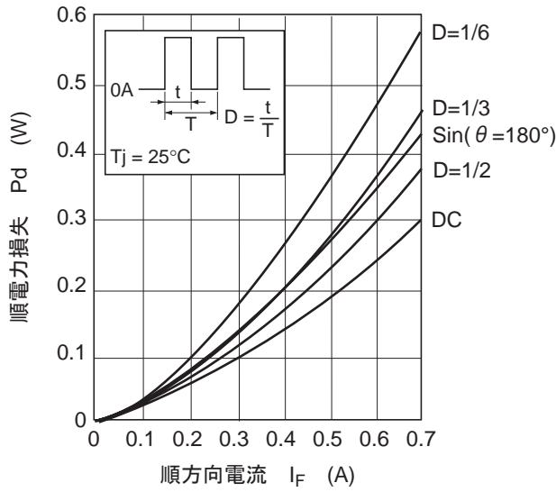
图4. 顺电力损失 对 顺电流特性
