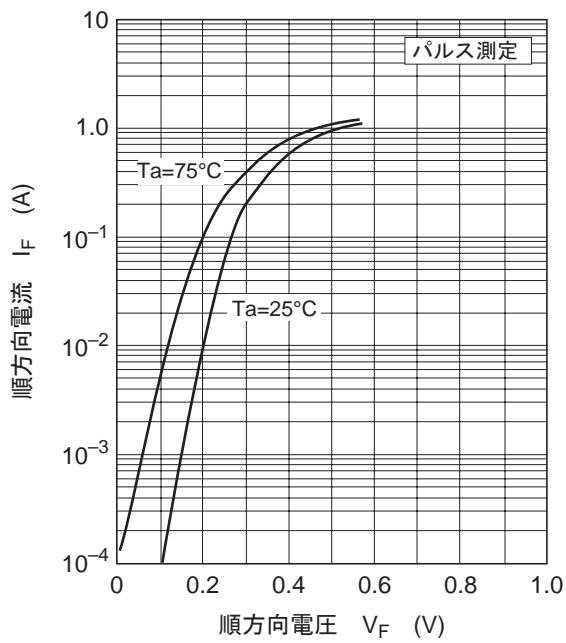
図1. 順方向特性
