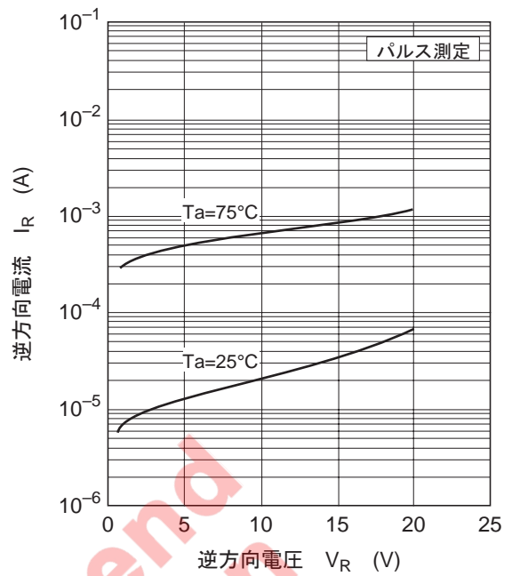
図2. 逆方向特性
