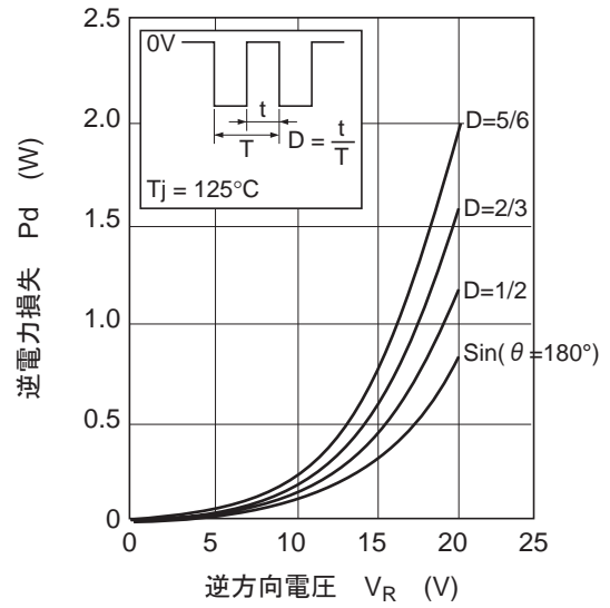
图5. 逆电力损失 对 逆电压特性
