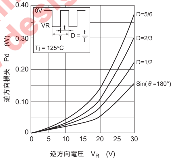
图4. 逆方向损失 对 逆电压特性
