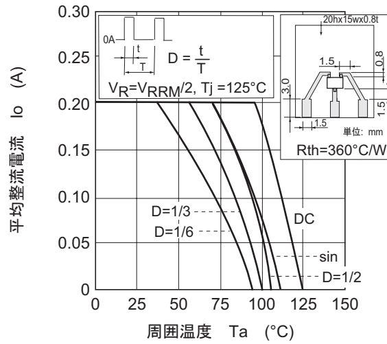
图5. 平均整流電流 对 周围温度特性
