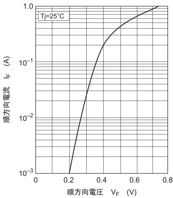
图1. 顺方向特性
