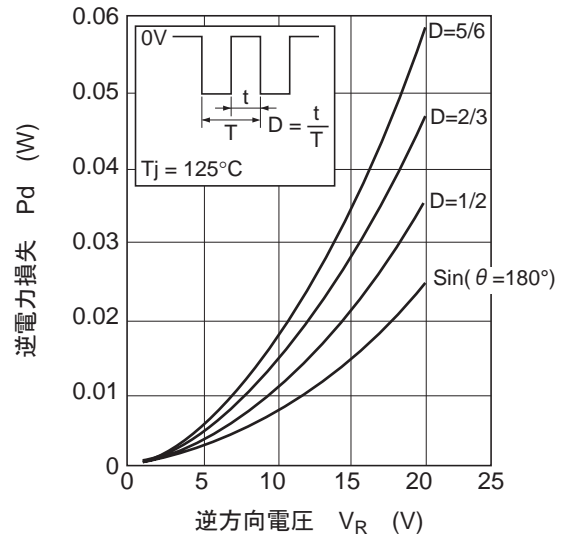
图5. 逆電力損失 对 逆電圧特性
