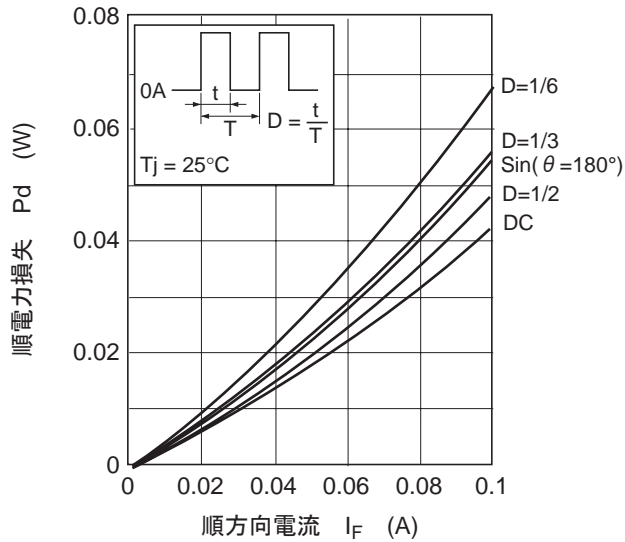
图4. 順電力損失 对 順電流特性
