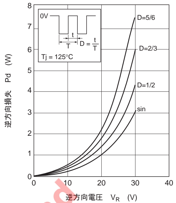
图5. 逆方向损失 对 逆电压特性
