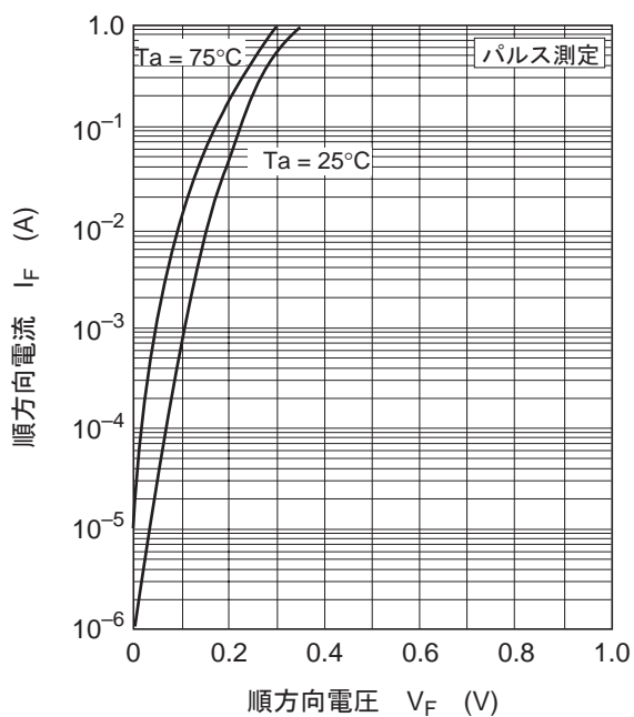
図1. 順方向特性
