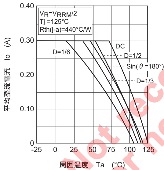
図6. 平均整流電流 対 周囲温度特性
