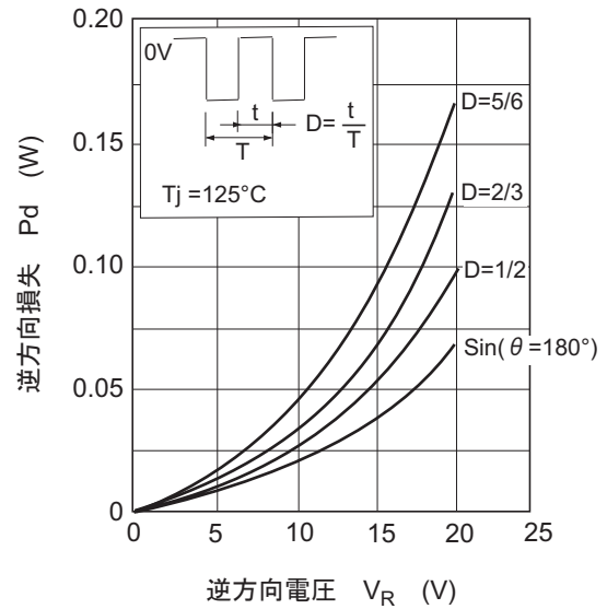
図5. 逆方向損失 対 逆電圧特性
