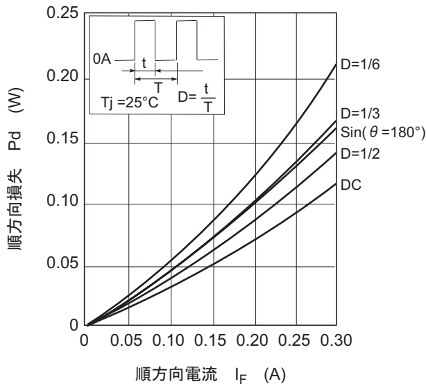
図4. 順方向損失 対 順電流特性
