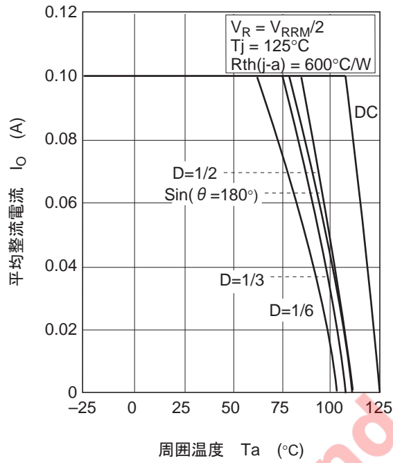
图5. 平均整流電流 对 周圍溫度特性
