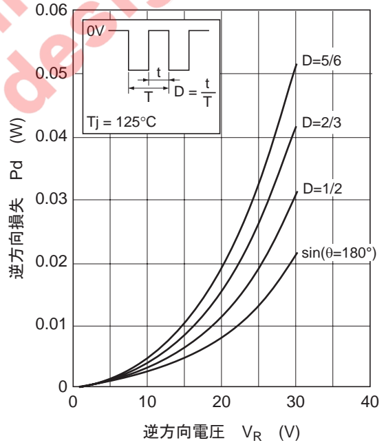
図4. 逆方向損失 対 逆電圧特性
