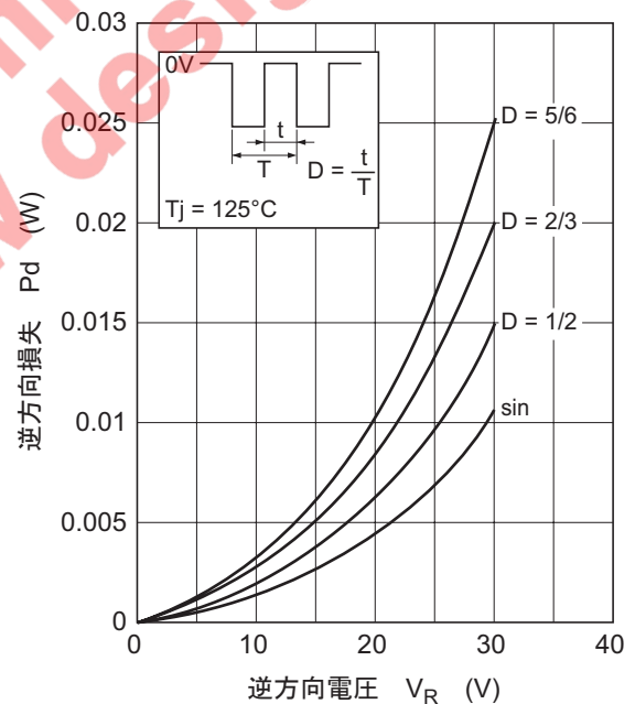
図4. 逆方向損失 対 逆方向電圧特性
