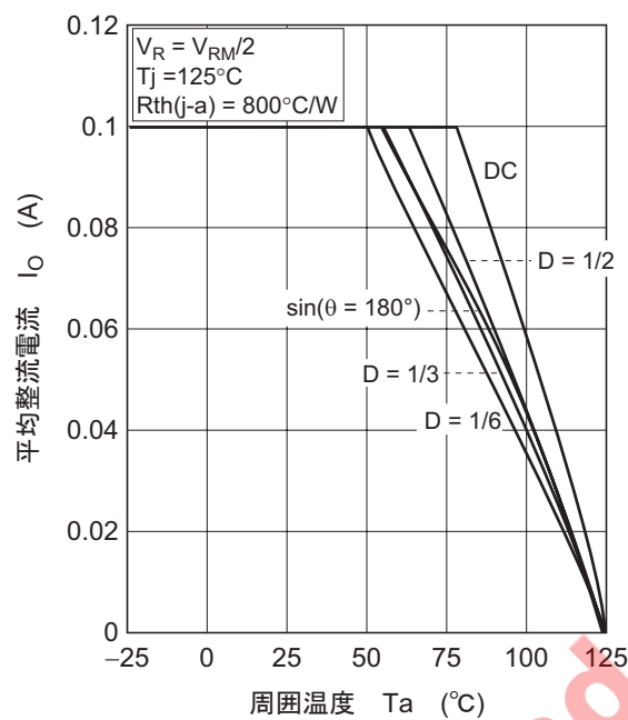
图5. 平均整流電流 对 周围温度特性
