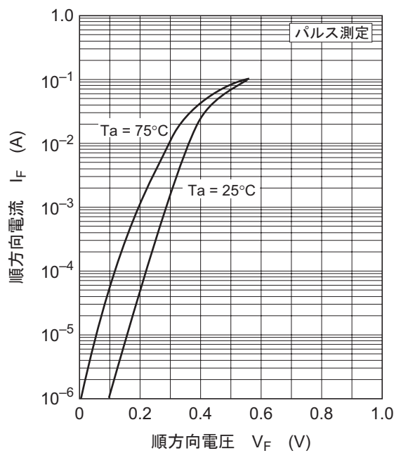
図1. 順方向特性
