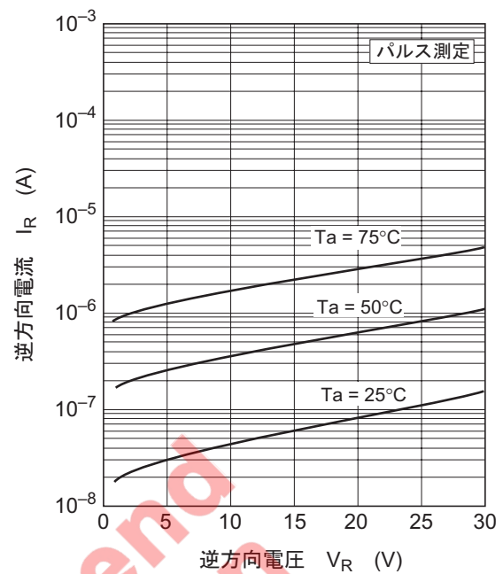
図2. 逆方向特性
