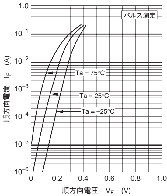
図1. 順方向特性
