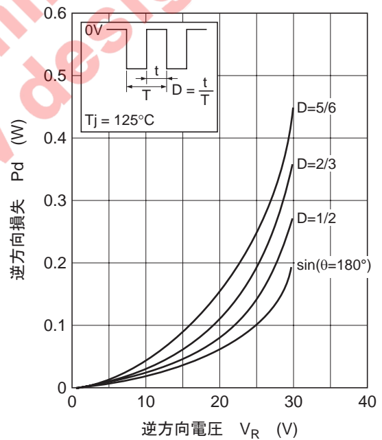
図4. 逆方向損失 対 逆方向電圧特性
