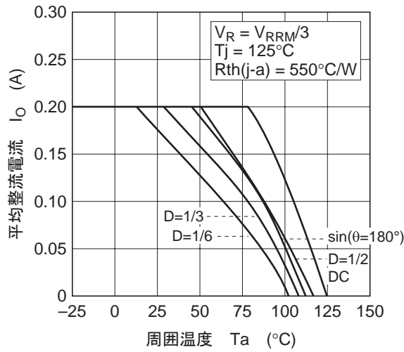
図5. 平均整流電流 対 周囲温度特性
