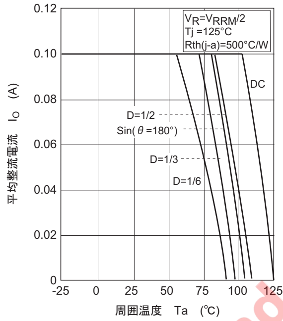
图5. 平均整流电流对周围温度特性
