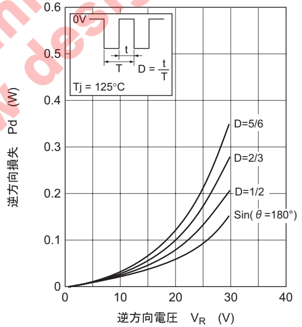
図4. 逆方向損失 対 逆方向電圧特性
