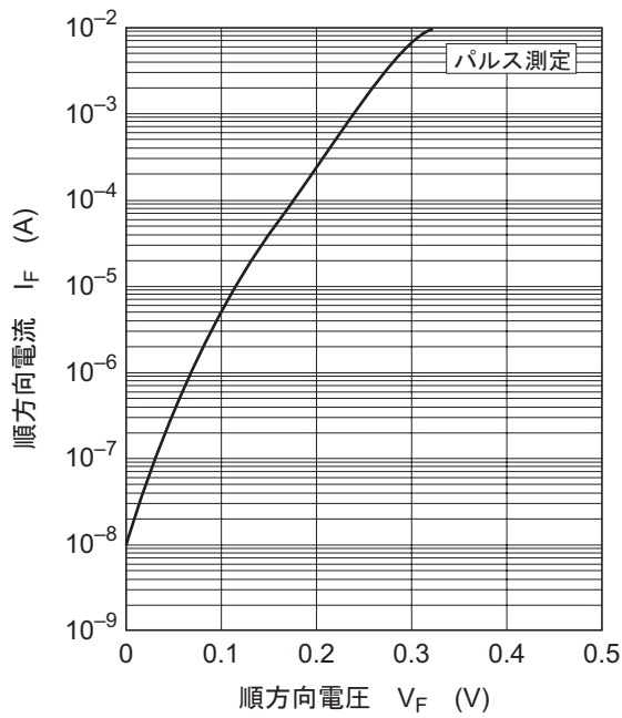
図1. 順方向特性
