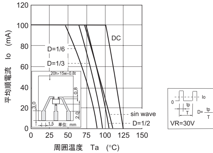
图5. 平均整流电流 对 周围温度特性
