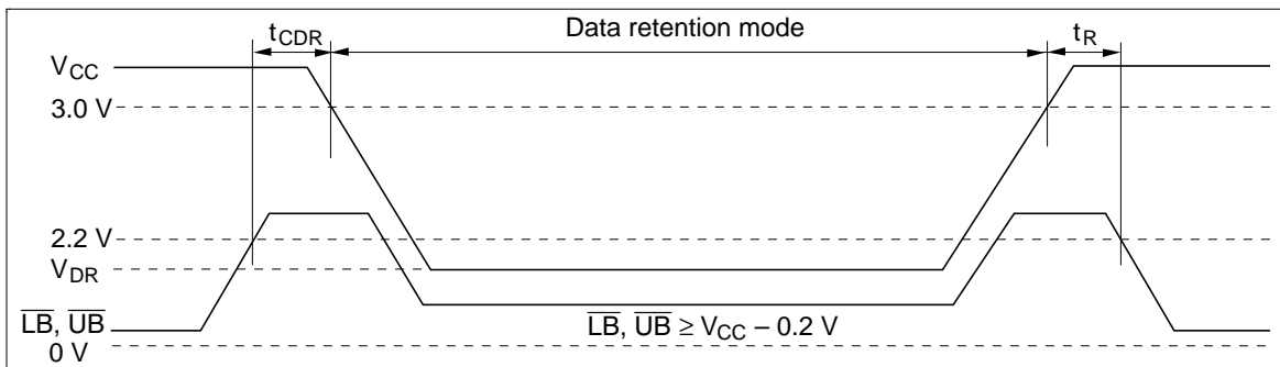
低電源電圧時データ保持タイミング波形(2) ( \overline{LB} , \overline{UB} Controlled)
