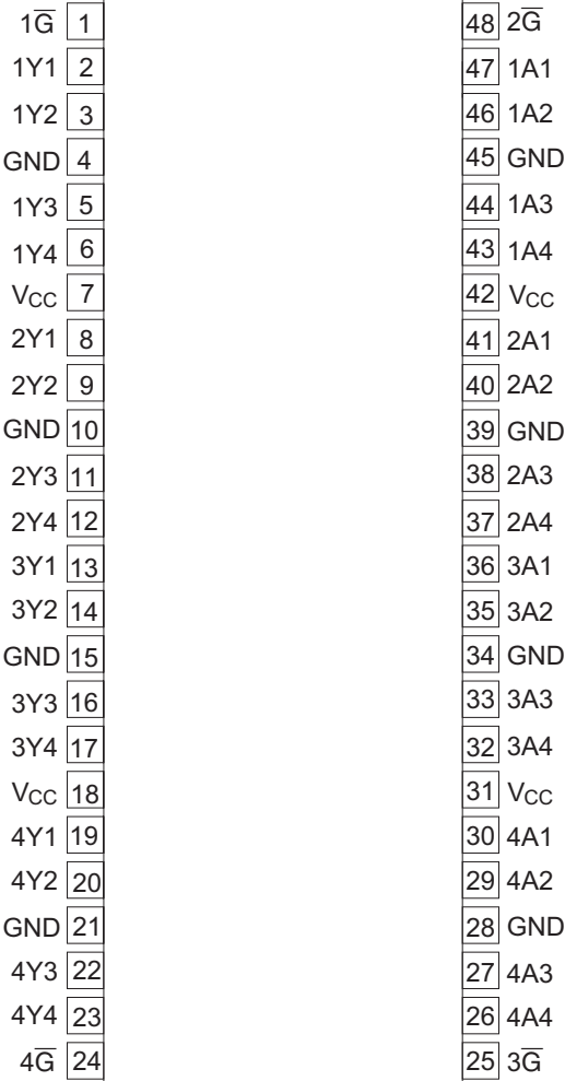
(上面図)
