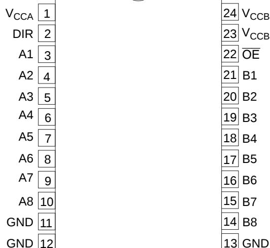
(上面図)
