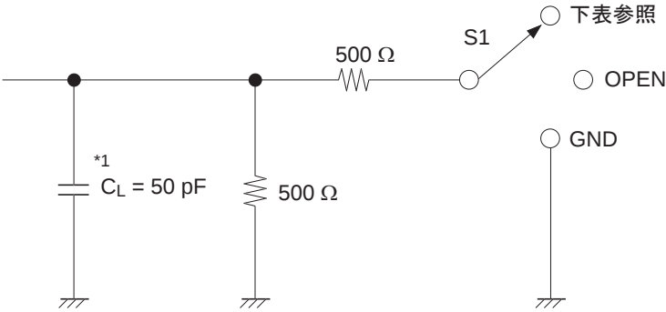
出力負荷回路
