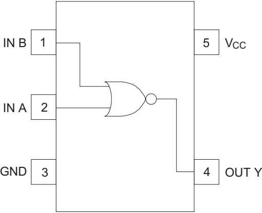
(上面図)
