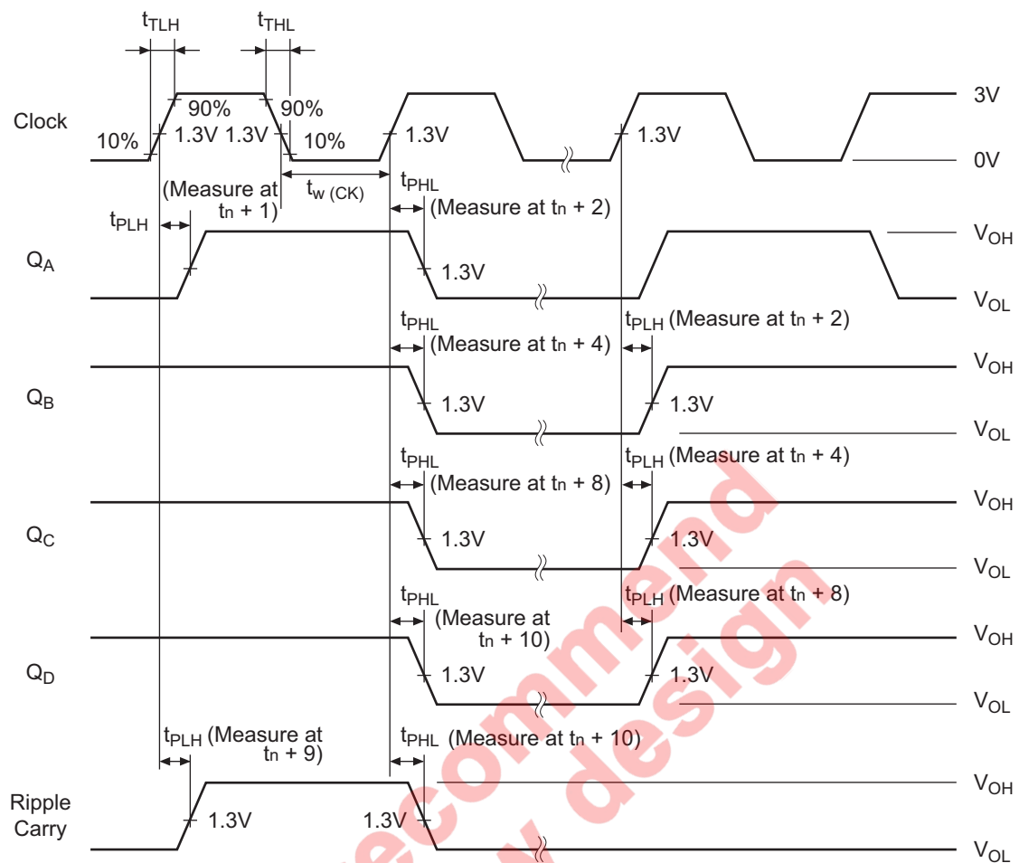
波形 1 f_{\max} , t_{PLH} , t_{PHL} , (Clock→Q, Ripple Carry)
