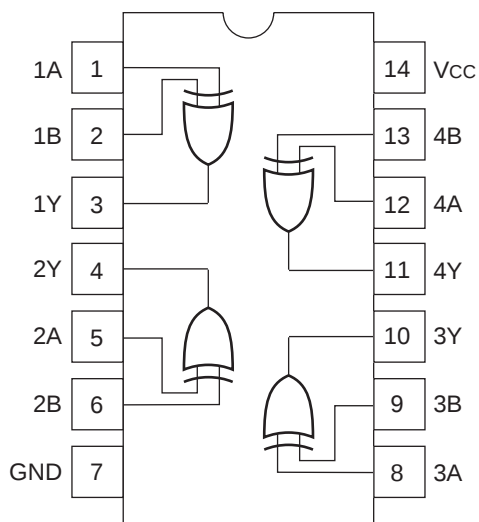
(上面図)
