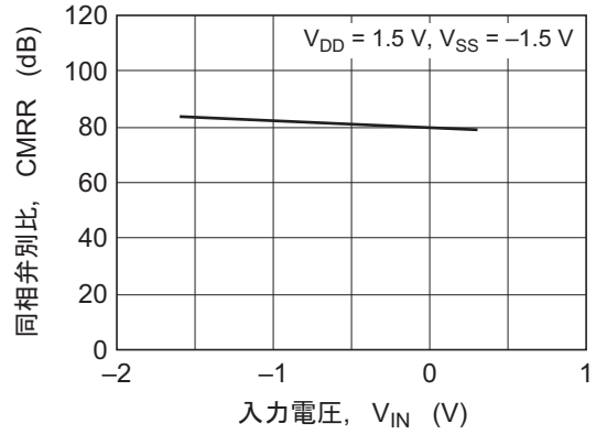
図14 HA1630S07 同相弁別比 対 入力電圧特性
