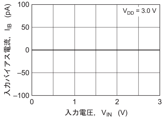
図16 HA1630S07 入力バイアス電流 対 入力電圧特性
