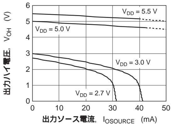
図5 HA1630S07 出力ハイ電圧 対 出力ソース電流特性
