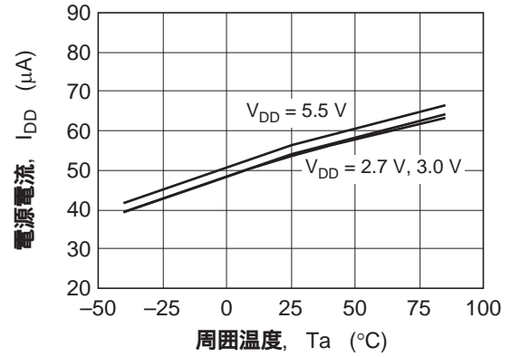
図2 HA1630S07 電源電流 対 周囲温度特性
