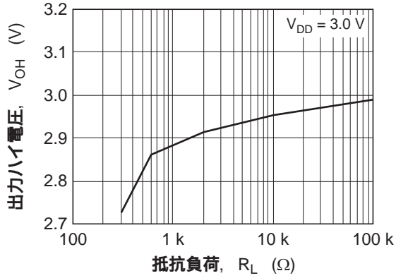
図3 HA1630S07 出力ハイ電圧 対 抵抗負荷特性
