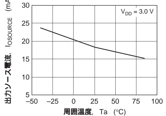
図6 HA1630S07 出力ソース電流 対 周囲温度特性
