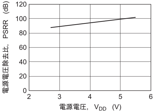
図15 HA1630S07 電源電圧除去比 対 電源電圧特性
