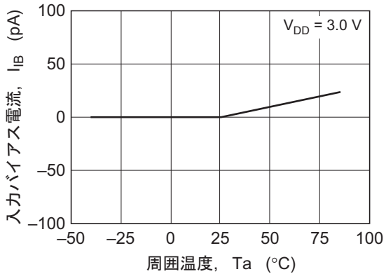
図17 HA1630S07 入力バイアス電流 対 周囲温度特性
