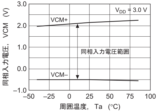
図13 HA1630S07 同相入力電圧 対 周囲温度特性
