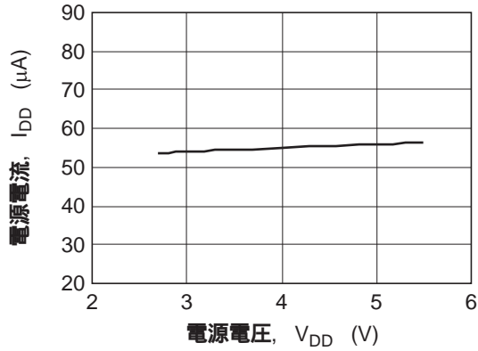
図1 HA1630S07 電源電流 対 電源電圧特性
