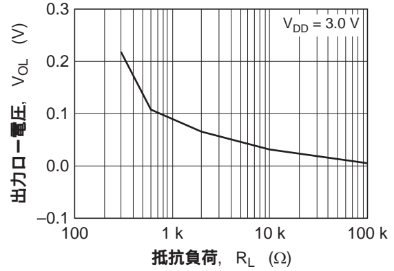
図4 HA1630S07 出力ロー電圧 対 抵抗負荷特性
