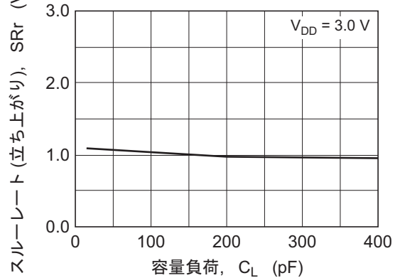
図18 HA1630S07 スルーレート (立ち上がり) 対 容量負荷特性
