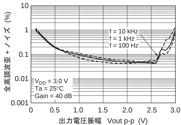
図 1-22. HA1630Q04 全高調波歪 + ノイズ 対 出力電圧振幅特性
