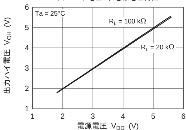
図 3-4. HA1630Q06 出力ハイ電圧 対 電源電圧特性
