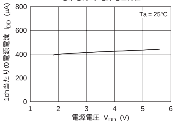
図 2-1. HA1630Q05 電源電流 対 電源電圧特性
