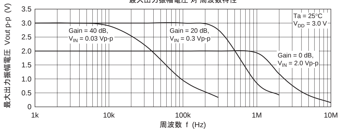
図 2-23. HA1630Q05 最大出力振幅電圧 対 周波数特性
