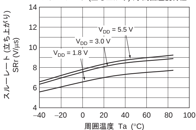
図 3-17. HA1630Q06 スルーレート (立ち上がり) 対 周囲温度特性
