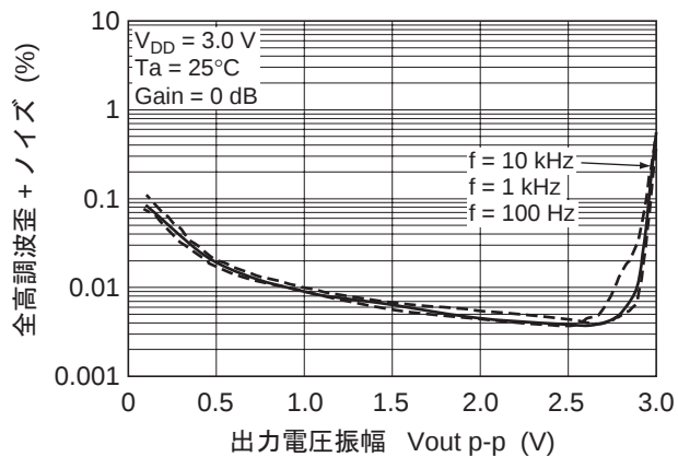
図 1-21. HA1630Q04 全高調波歪 + ノイズ 対 出力電圧振幅特性
