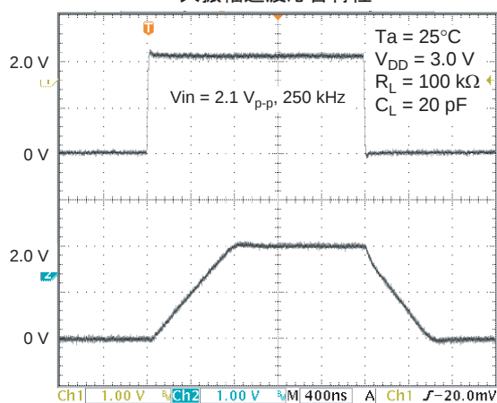
図 1-19. HA1630Q04 大振幅過渡応答特性
