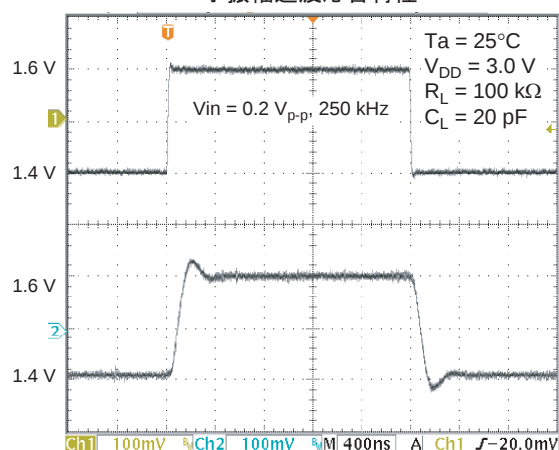
図 1-20. HA1630Q04 小振幅過渡応答特性
