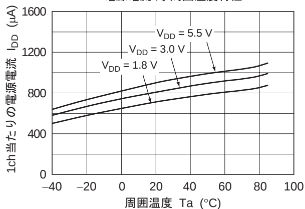
図 3-2. HA1630Q06 電源電流 対 周囲温度特性
