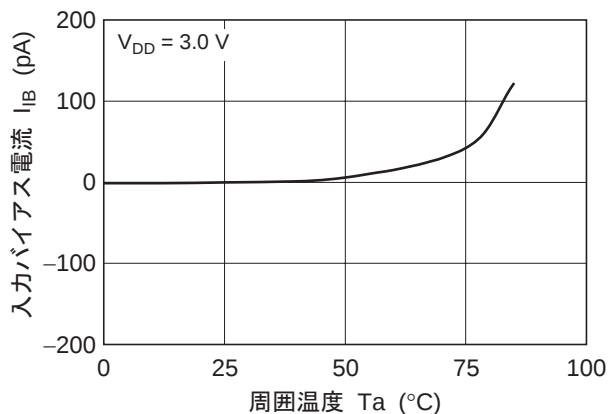
図 1-15. HA1630Q04 入力バイアス電流 対 周囲温度特性
