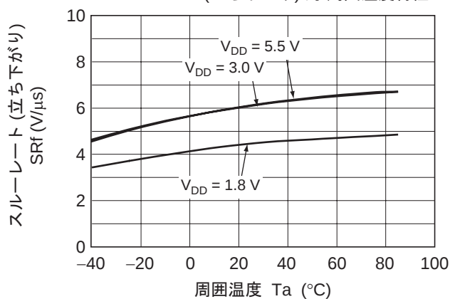
図 2-18. HA1630Q05 スルーレート (立ち下がり) 対 周囲温度特性
