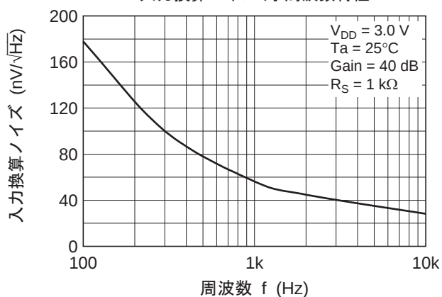
図 2-24. HA1630Q05 入力換算ノイズ 対 周波数特性
