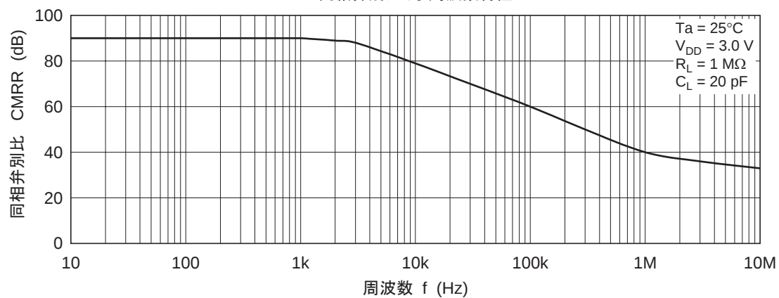
図 2-13. HA1630Q05 同相弁別比 対 周波数特性
