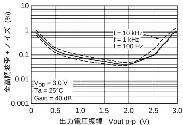
図 3-23. HA1630Q06
