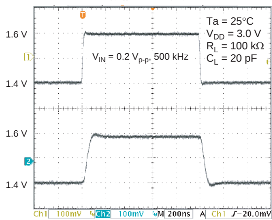
図 3-20. HA1630Q06 小振幅過渡応答特性
