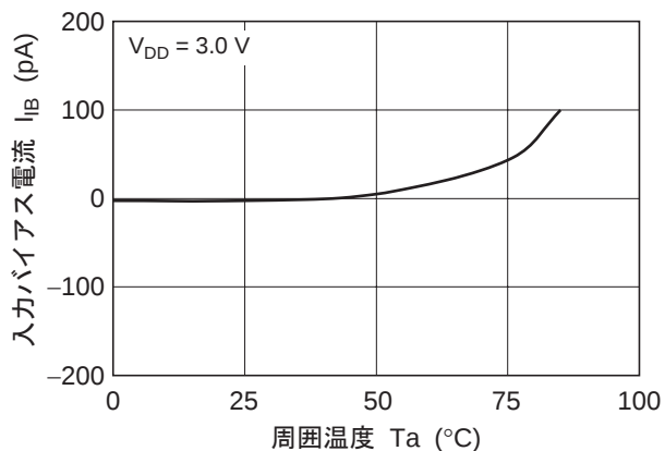
図 2-15. HA1630Q05 入力バイアス電流 対 周囲温度特性
