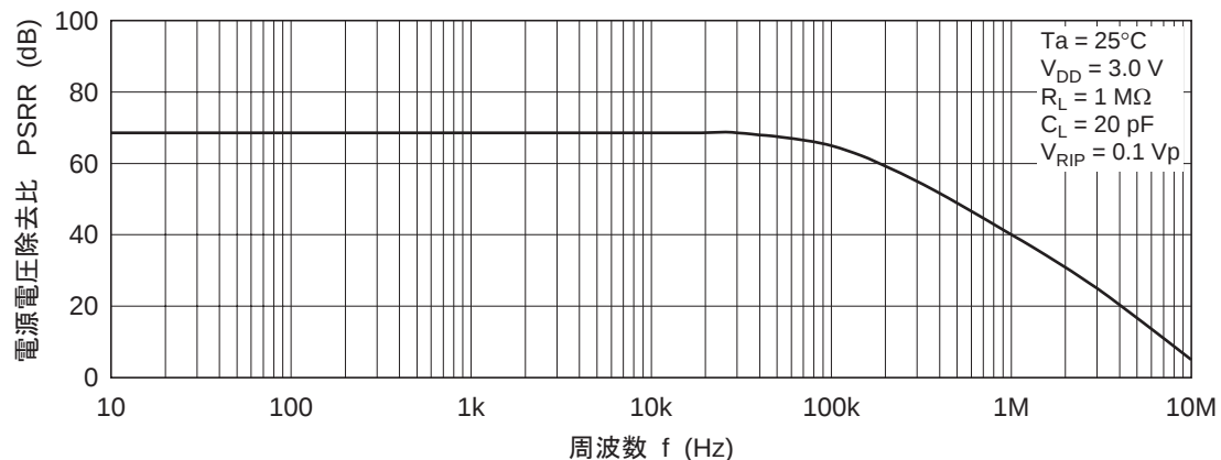
図 3-12. HA1630Q06 電源電圧除去比 対 周波数特性
