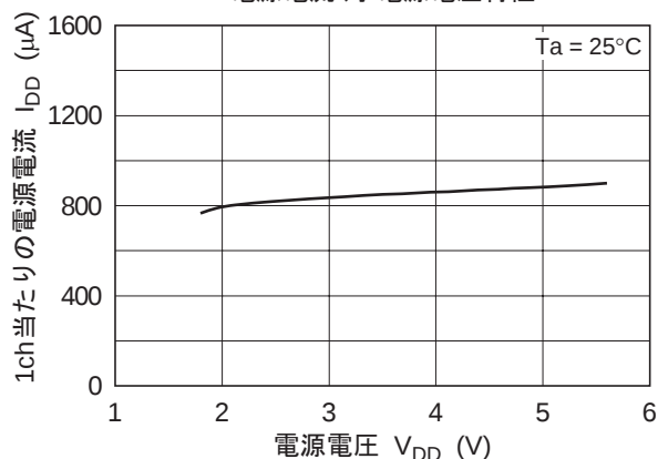
図 3-1. HA1630Q06 電源電流 対 電源電圧特性
