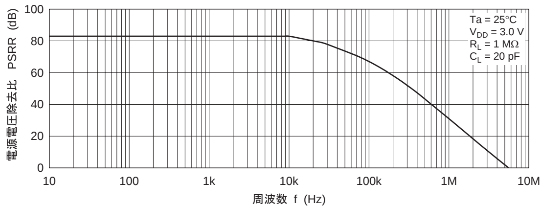
図 1-12. HA1630Q04 電源電圧除去比 対 周波数特性
