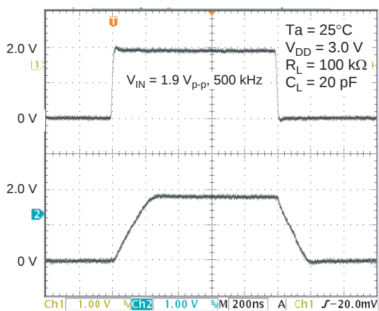
図 3-19. HA1630Q06 大振幅過渡応答特性
