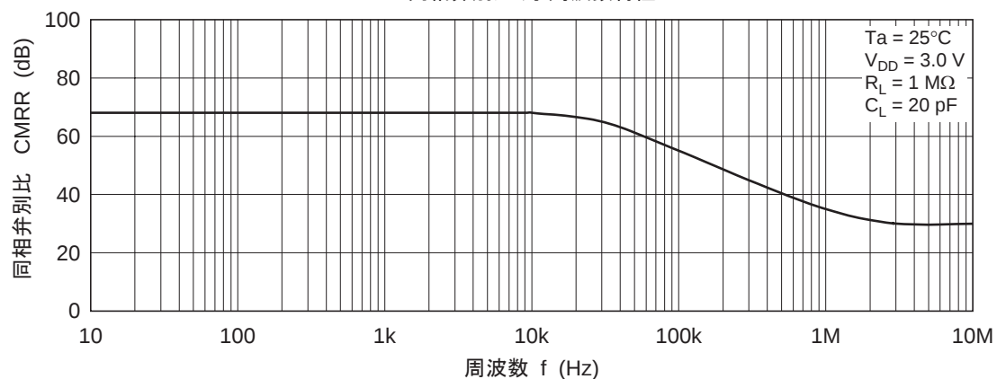
図 3-13. HA1630Q06 同相弁別比 対 周波数特性
