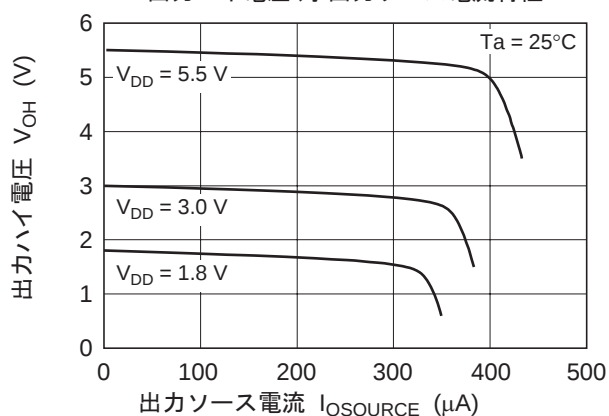
図 2-3. HA1630Q05 出力ハイ電圧 対 出力ソース電流特性
