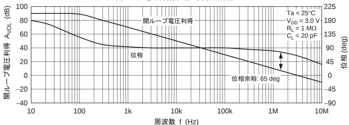
図 3-14. HA1630Q06 開ループ電圧利得, 位相 対 周波数特性
