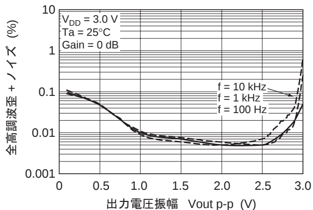
図 3-21. HA1630Q06
