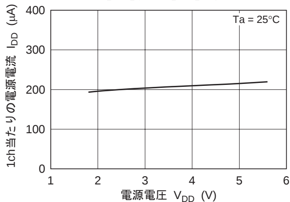
図 1-1. HA1630Q04 電源電流 対 電源電圧特性
