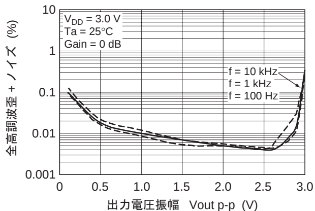
図 2-21. HA1630Q05 全高調波歪 + ノイズ 対 出力電圧振幅特性
