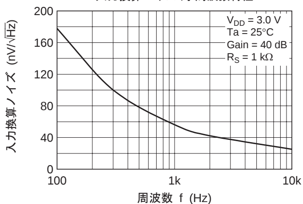
図 3-24. HA1630Q06
