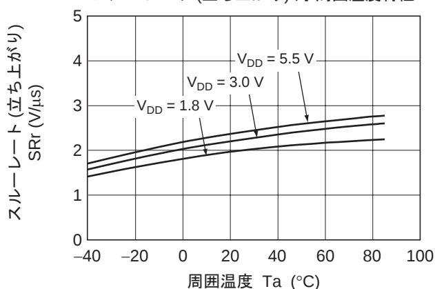
図 1-17. HA1630Q04 スルーレート (立ち上がり) 対 周囲温度特性
