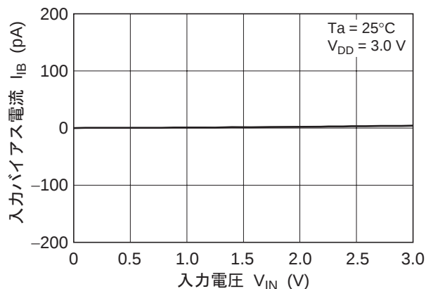
図 2-16. HA1630Q05 入力バイアス電流 対 入力電圧特性
