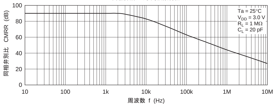
図 1-13. HA1630Q04 同相弁別比 対 周波数特性
