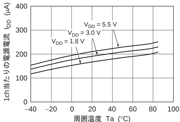
図 1-2. HA1630Q04 電源電流 対 周囲温度特性
