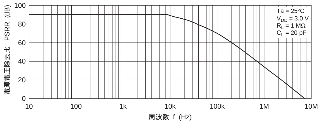
図 2-12. HA1630Q05 電源電圧除去比 対 周波数特性
