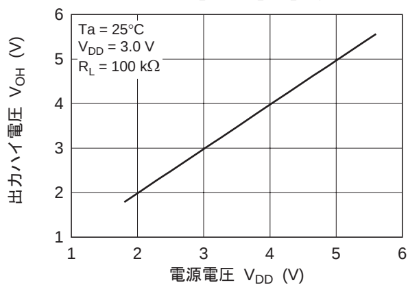
図 1-4. HA1630Q04 出力ハイ電圧 対 電源電圧特性
