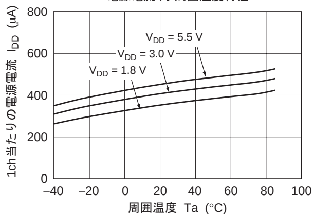
図 2-2. HA1630Q05 電源電流 対 周囲温度特性
