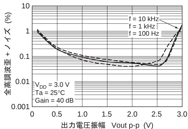
図 2-22. HA1630Q05 全高調波歪 + ノイズ 対 出力電圧振幅特性
