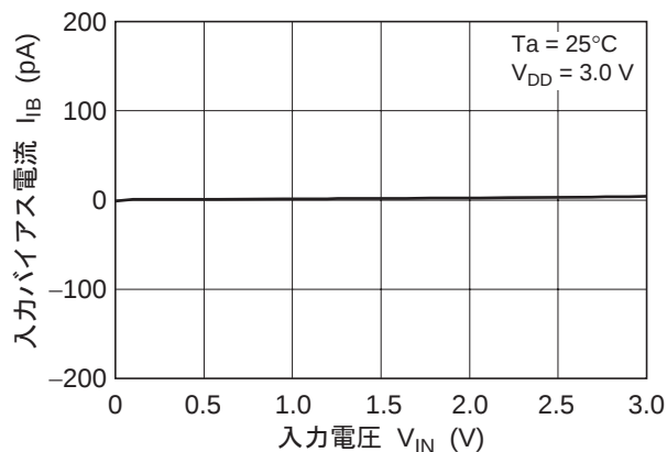
図 3-16. HA1630Q06 入力バイアス電流 対 入力電圧特性
