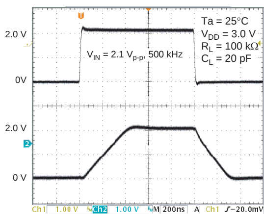
図 2-19. HA1630Q05 大振幅過渡応答特性
