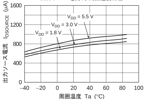
図 3-5. HA1630Q06 出力ソース電流 対 周囲温度特性
