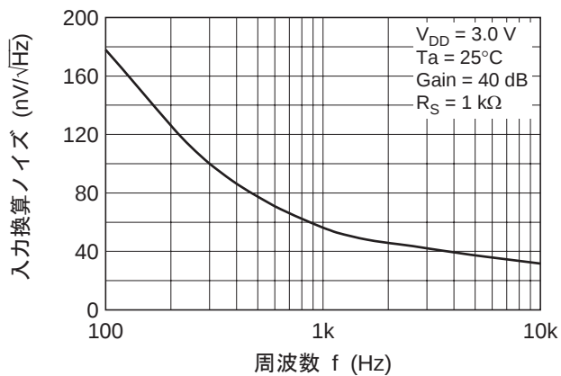
図 1-24. HA1630Q04 入力換算ノイズ 対 周波数特性
