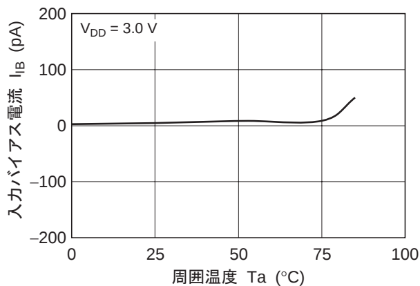
図 3-15. HA1630Q06 入力バイアス電流 対 周囲温度特性
