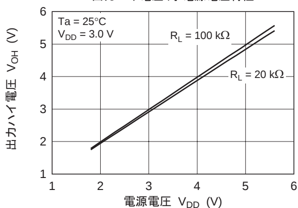
図 2-4. HA1630Q05 出力ハイ電圧 対 電源電圧特性
