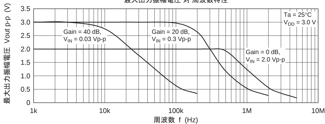
図 1-23. HA1630Q04 最大出力振幅電圧 対 周波数特性
