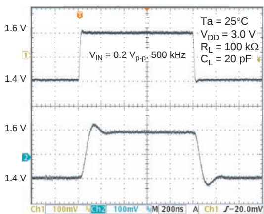
図 2-20. HA1630Q05 小振幅過渡応答特性
