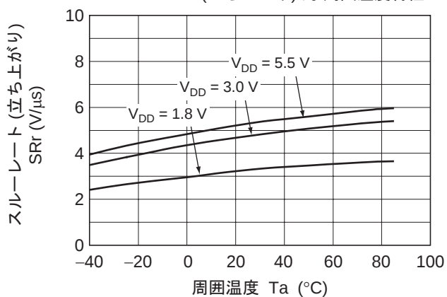
図 2-17. HA1630Q05 スルーレート (立ち上がり) 対 周囲温度特性
