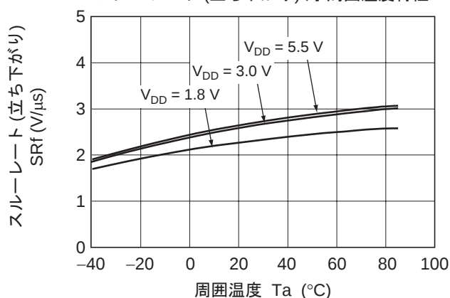
図 1-18. HA1630Q04 スルーレート (立ち下がり) 対 周囲温度特性
