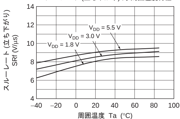
図 3-18. HA1630Q06 スルーレート (立ち下がり) 対 周囲温度特性
