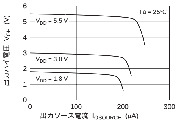
図 1-3. HA1630Q04 出力ハイ電圧 対 出力ソース電流特性
