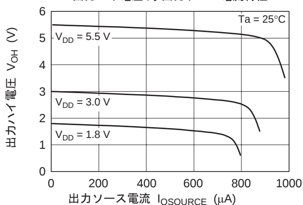
図 3-3. HA1630Q06 出力ハイ電圧 対 出力ソース電流特性
