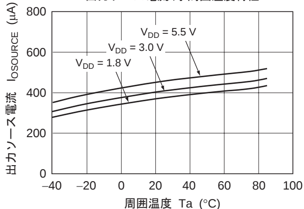
図 2-5. HA1630Q05 出力ソース電流 対 周囲温度特性
