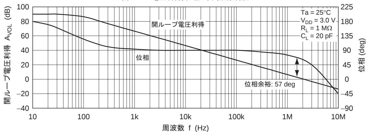
図 1-14. HA1630Q04 開ループ電圧利得, 位相 対 周波数特性
