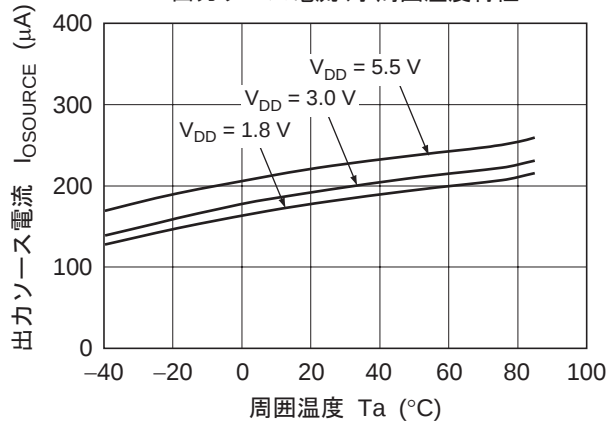
図 1-5. HA1630Q04 出力ソース電流 対 周囲温度特性
