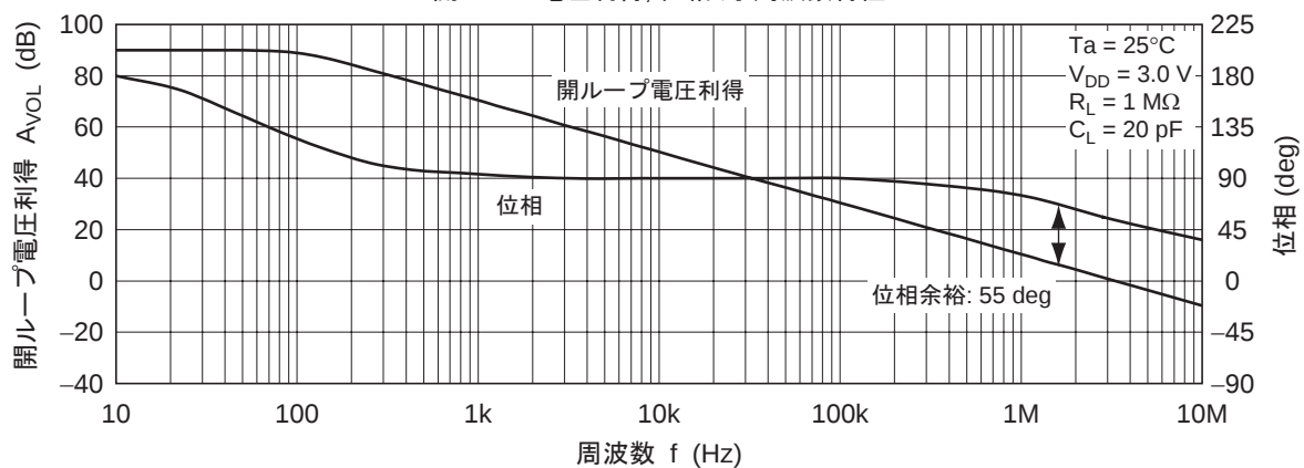
図 2-14. HA1630Q05 開ループ電圧利得, 位相 対 周波数特性
